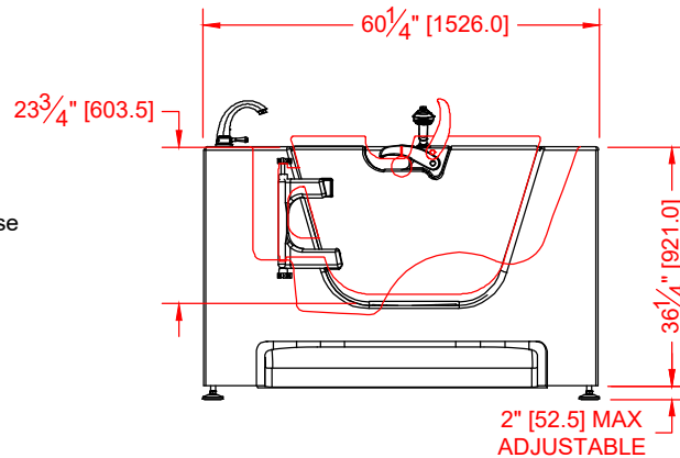
FRONT ELEVATION - SCALE: \frac{3}{8} " = 1'-0"
